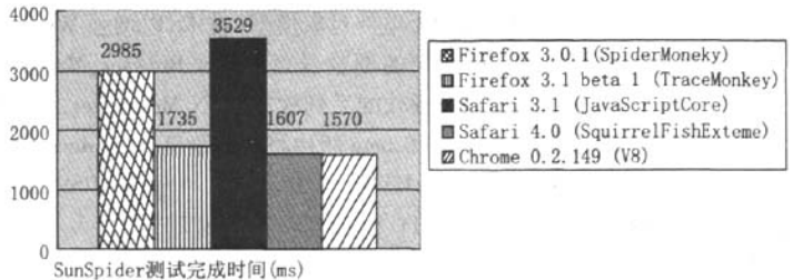
图 4 不同 JavaScript 引擎的性能对比
