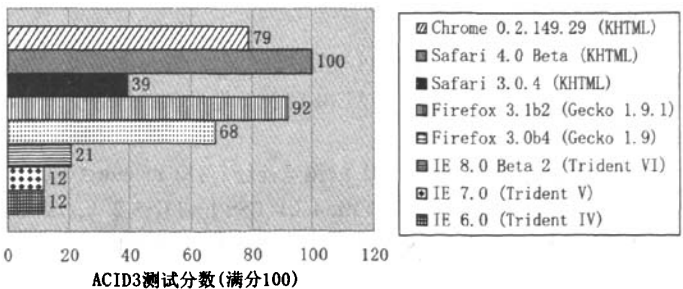
图 5 不同排版引擎的性能对比
