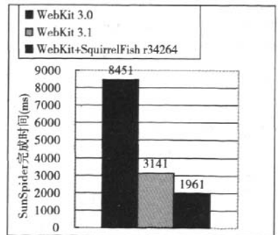
图 2 SquirrelFish 与 JavaScriptCore 的性能对比
