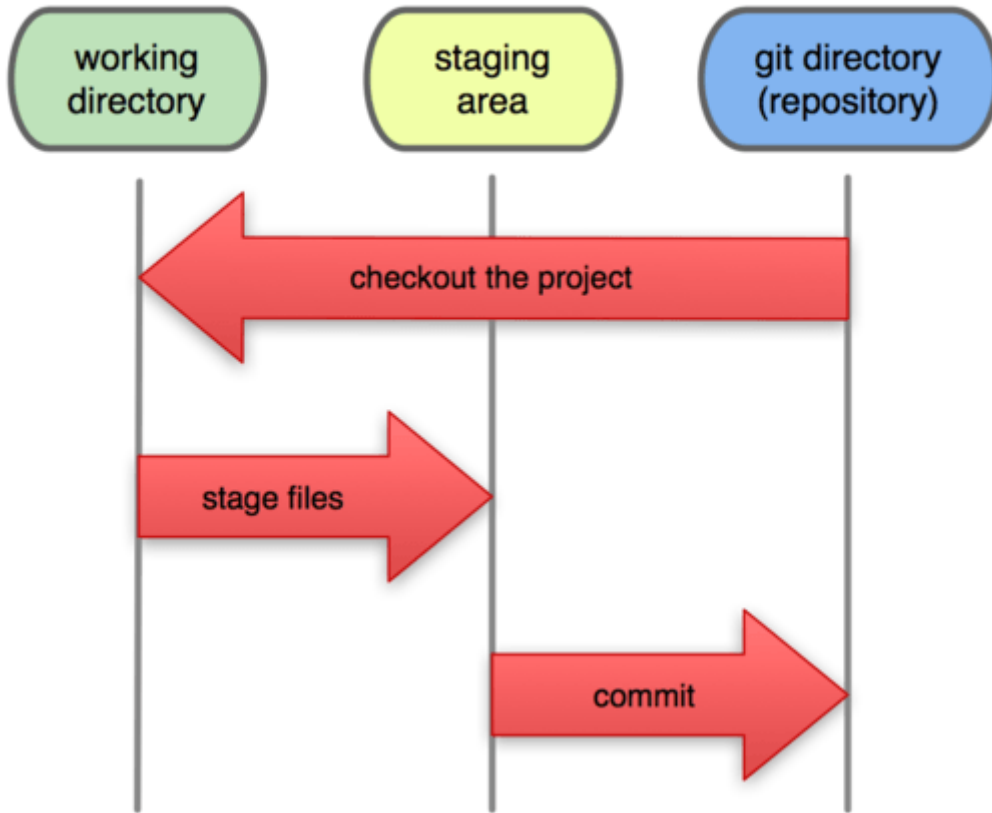
图 1-6. 工作目录，暂存区域，以及本地仓库
