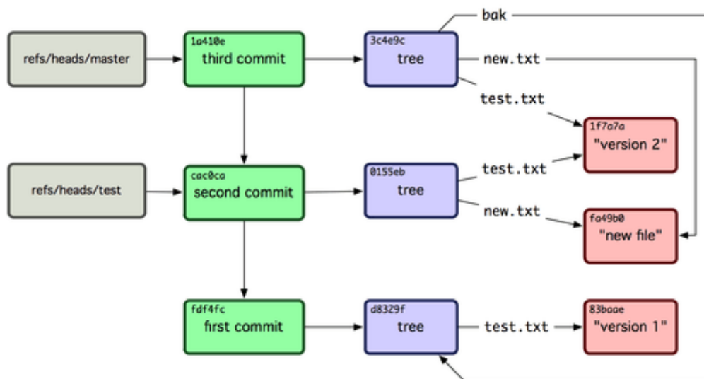
图 9-4. 包含分支引用的 Git 目录对象
