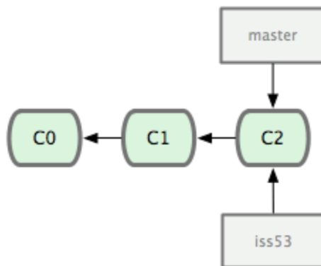
图 3-11. 创建了一个新分支的指针
