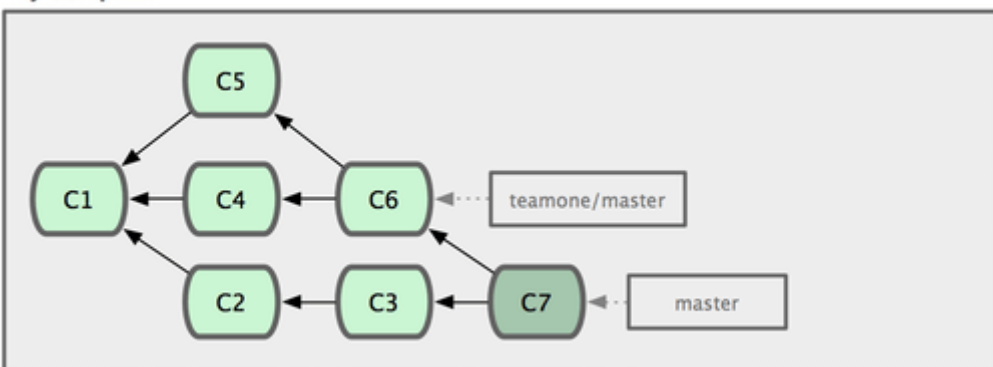
图 3-37. 抓取他人提交，并入自己主干。
