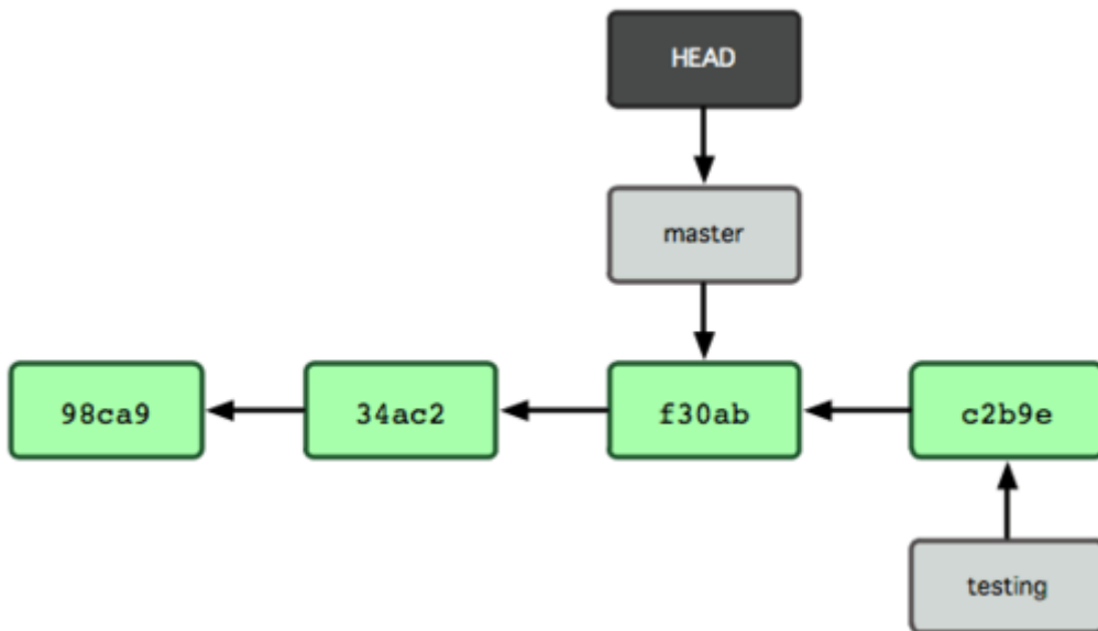
图 3-8. HEAD 在一次 checkout 之后移动到了另一个分支 这条命令做了两件事。它把 HEAD 指针移回到 master 分支，并把工作目录中的文件换成了 master 分支所指向的快照内容。也就是说，现在开始所做的改动，将始于本项目中一个较老的版本。它的主要作用是将 testing 分支里作出的修改暂时取消，这样你就可以向另一个方向进行开发。
