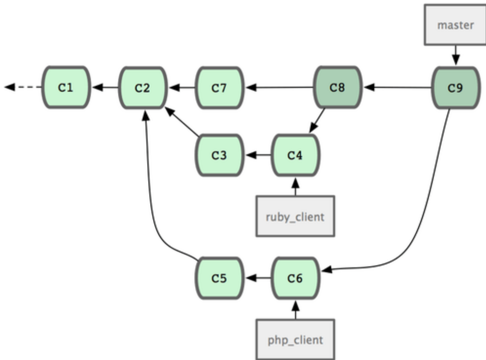
图 5-20. 合并特性分支之后
