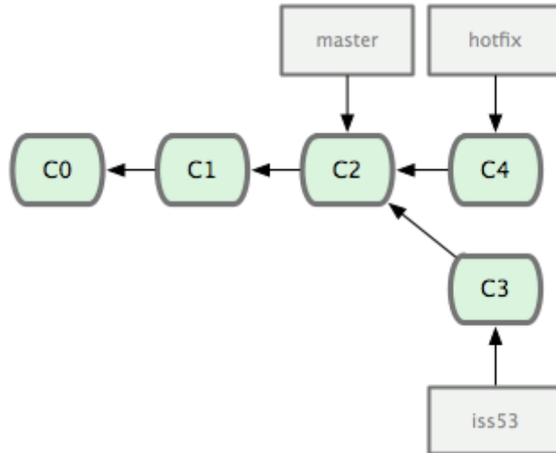
图 3-13. hotfix 分支是从 master 分支所在点分化出来的 有必要作些测试，确保修补是成功的，然后回到 master 分支并把它合并进来，然后发布到生产服务器。用 git merge 命令来进行合并：
