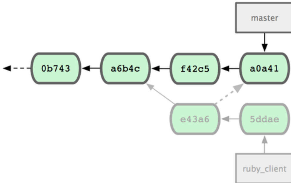
图 5-27. 挑拣 (cherry-pick) 之后的历史 现在，你可以删除这个特性分支并丢弃你不想引入的那些 commit。
