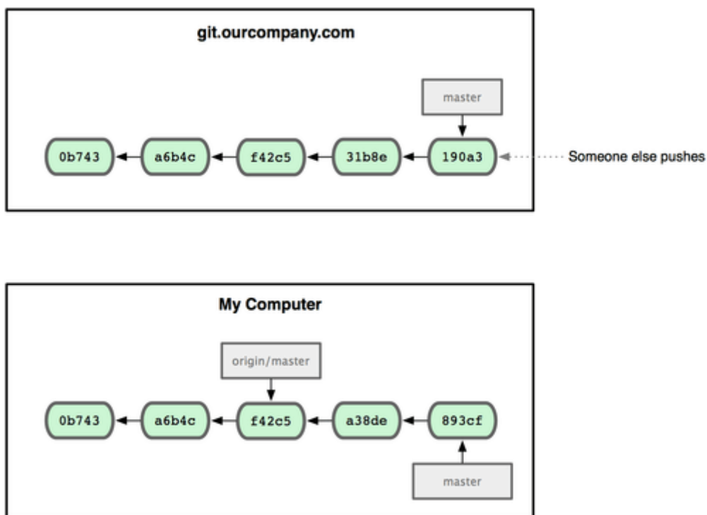
图 3-23. 在本地工作的同时有人向远程仓库推送内容会让提交历史开始分流。可以运行 git fetch origin 来同步远程服务器上的数据到本地。该命令首先找到 origin 是哪个服务器（本例为 git.ourcompany.com ），从上面获取你尚未拥有的数据，更新你本地的数据库，然后把 origin/master 的指针移到它最新的位置上（见图 3-24）。
