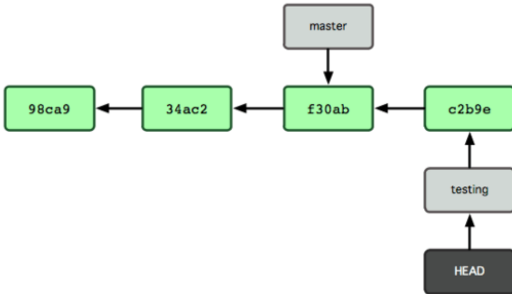
图 3-7. 每次提交后 HEAD 随着分支一起向前移动 非常有趣，现在 testing 分支向前移动了一格，而 master 分支仍然指向原先 git checkout 时所在的 commit 对象。现在我们回到 master 分支看看：
