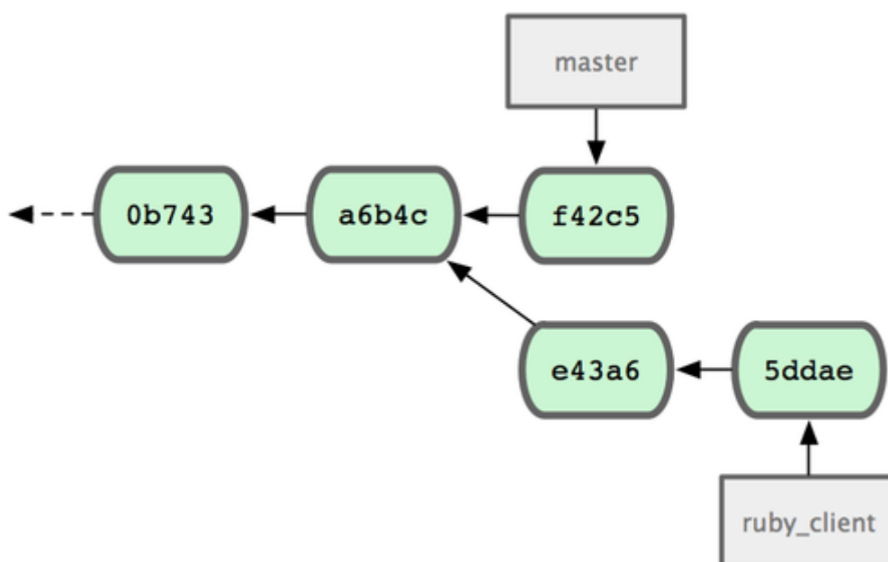
图 5-26. 挑拣（cherry-pick）之前的历史
