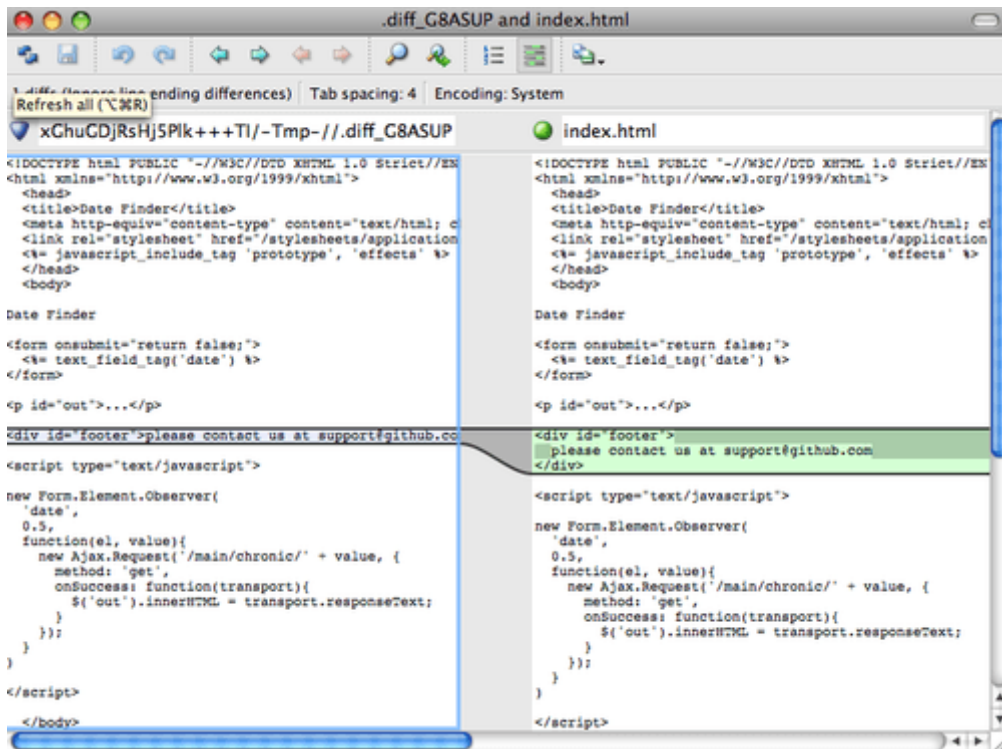
图 7-1. P4Merge.
