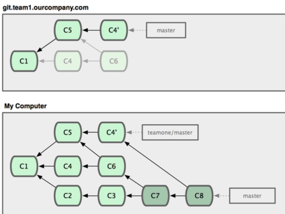
图 3-38. 有人推送了衍合后得到的 C4'，丢弃了你作为开发基础的 C4 和 C6。下载更新后需要合并，但此时衍合产生的提交对象 C4' 的 SHA-1 校验值和之前 C4 完全不同，所以 Git 会把它们当作新的提交对象处理，而实际上此刻你的提交历史 C7 中早已经包含了 C4 的修改内容，于是合并操作会把 C7 和 C4' 合并为 C8（见图 3-39）：
