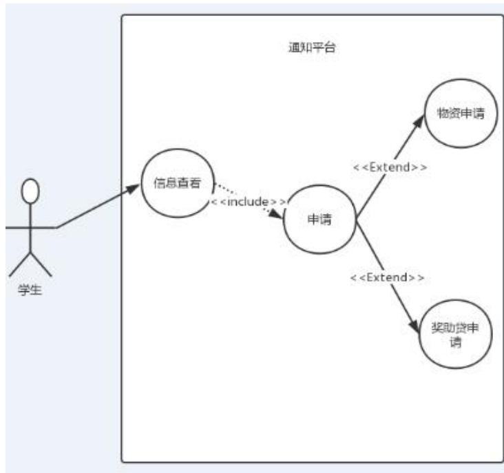
图 3-10 通知平台使用用例图
