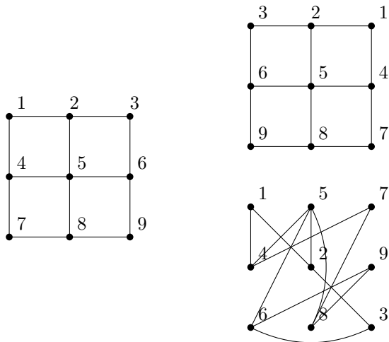
图 9.2: “田” 的对称性
