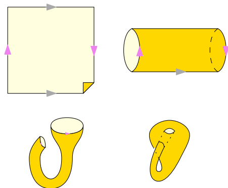
图 6.6: Klein 瓶
