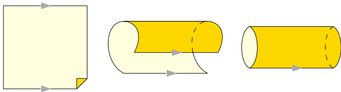
图 6.3: “管子”
