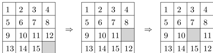
图 9.4: 15 拼板问题
