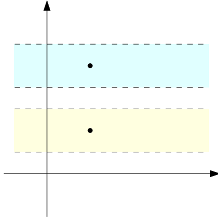
图 7.6: T2 的乘性
