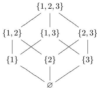
图 13.1: 2^{\{1,2,3\}} 的 Hasse 图
