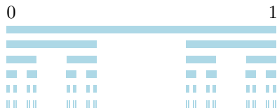
图 3.5: Cantor 集
