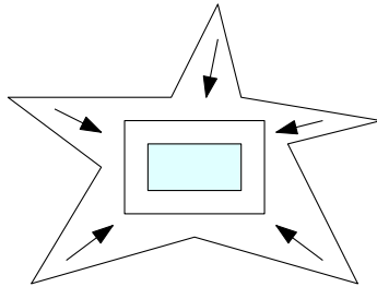
图 7.7: T3 的乘性
