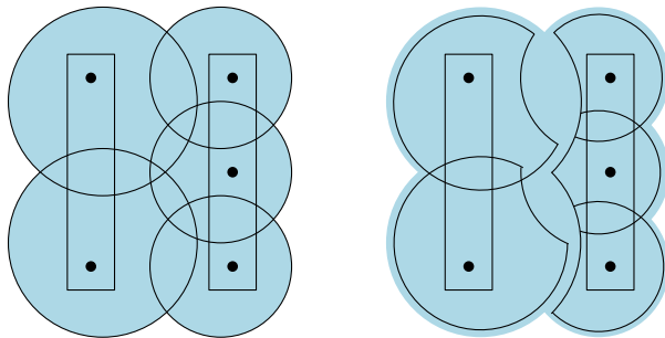
图 7.9: Lindelöf 定理
