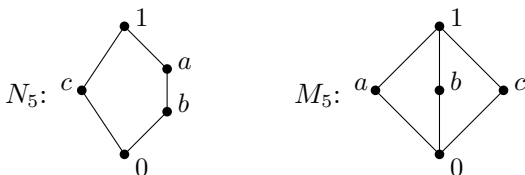
图 14.3: N_5 和 M_5
