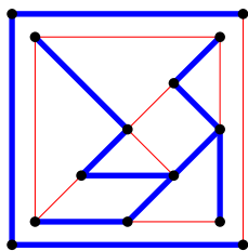
图 5.5: 支撑森林
