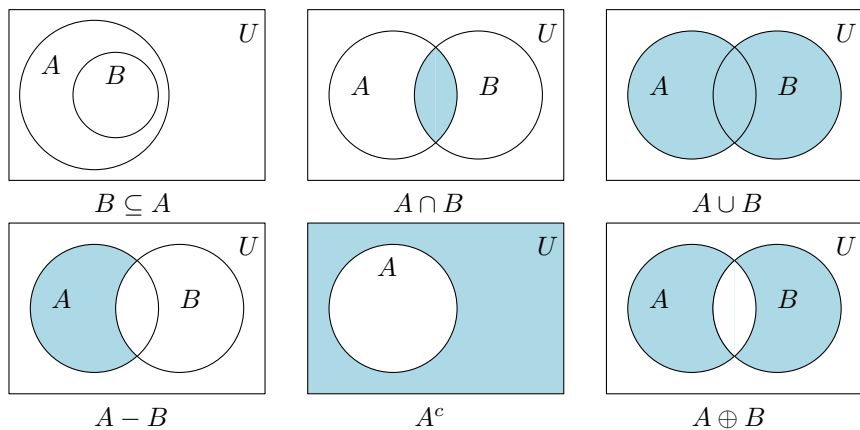
图 1.1: Venn 图
