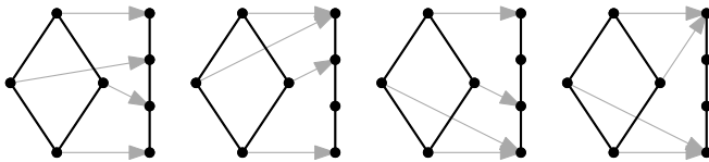
图 13.7: 格的同态
