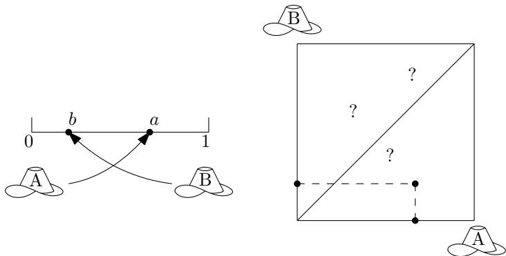
图 12.1: 飞镖游戏
