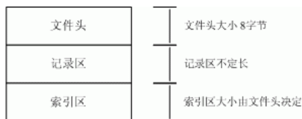
图1. QQWry.dat文件结构
