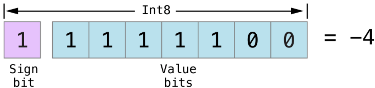
图片 2.40 Art/bitshiftSignedMinusFour_2x.png
