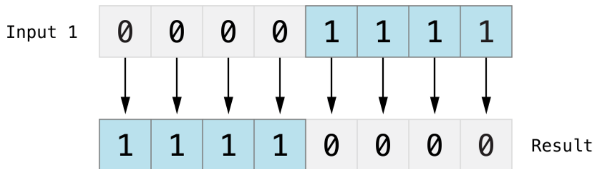
图片 2.34 Art/bitwiseNOT_2x.png
