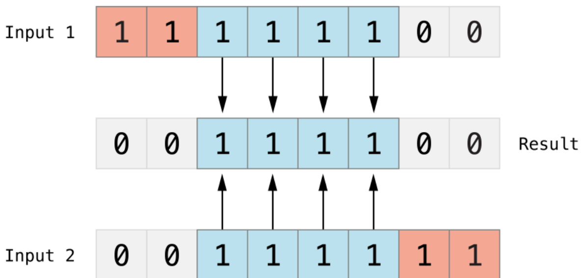
图片 2.35 Art/bitwiseAND_2x.png
