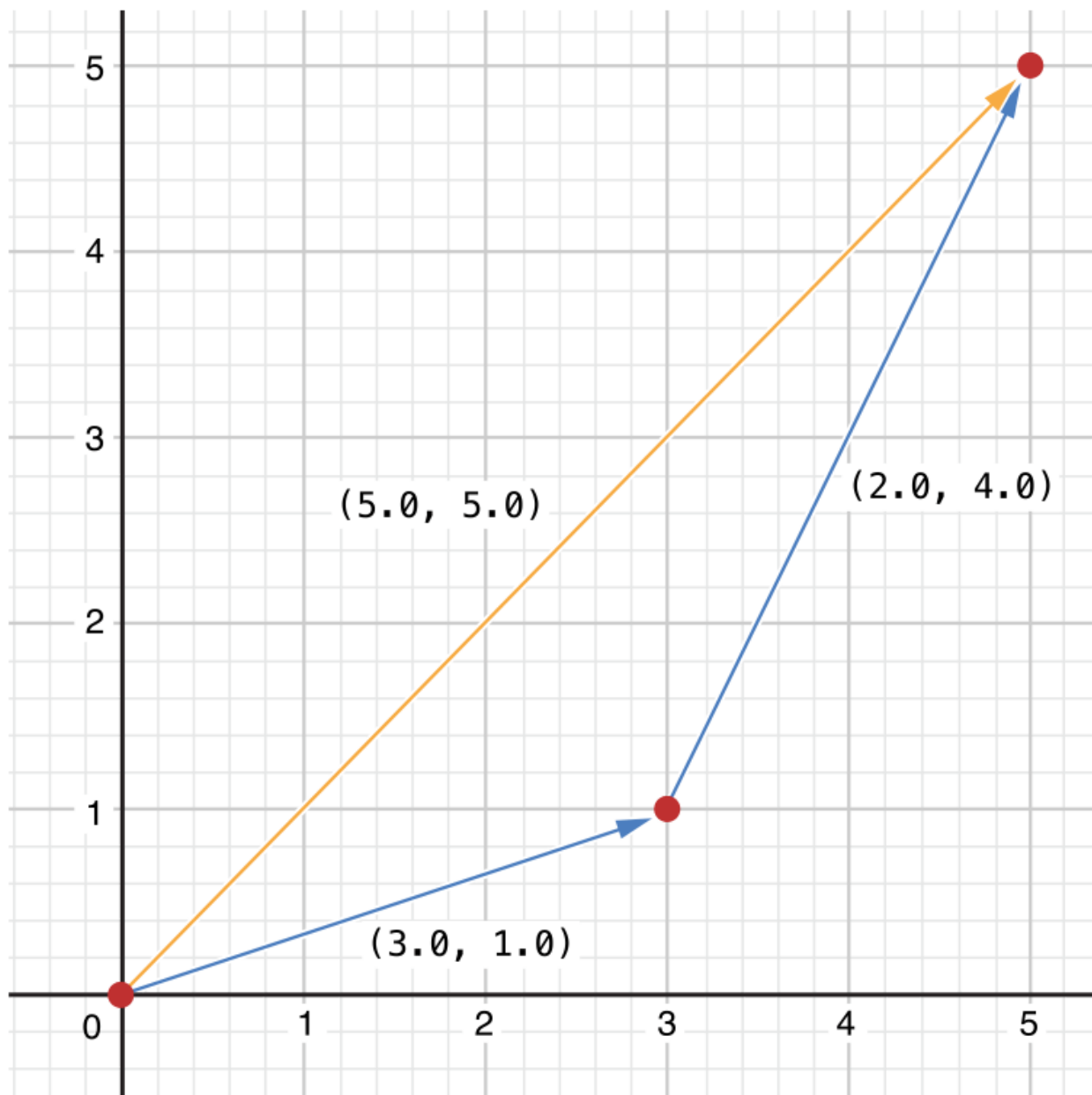
图片 2.47 Art/vectorAddition_2x.png
