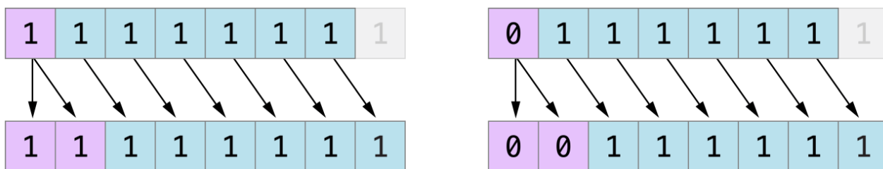
图片 2.43 Art/bitshiftSigned_2x.png
